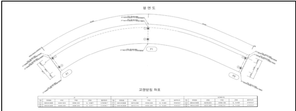
【그림 17.3.1】 교량받침 배치도
