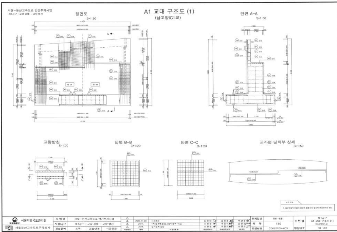
【그림 17.1.6】 교대 일반도 및 구조도
