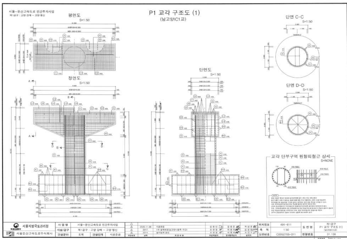
【그림 17.1.7】 교각 일반도 및 구조도
